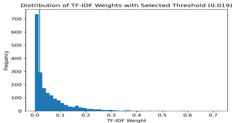
شکل ۳. نمودار توزیع وزن‌های TF-IDF و تعیین آستانه برش واژگان.
