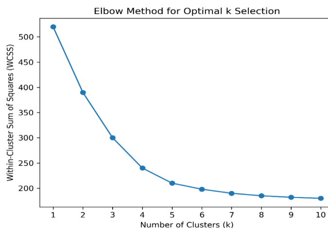
شکل ۴. تعیین تعداد بهینه خوشه‌ها به روش Elbow.
